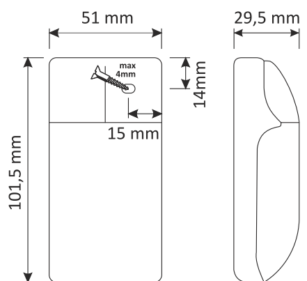
Gehäusemaße
