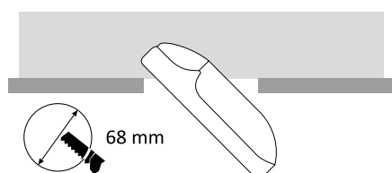
Deckenmontage
