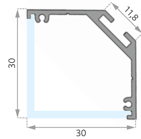
ANGOLO ECK-PROFIL 30×30 mm
